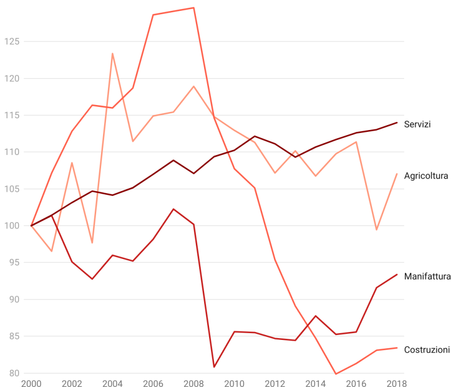
Grafico 1. PRODUZIONE. NUMERO INDICE 2000=100
