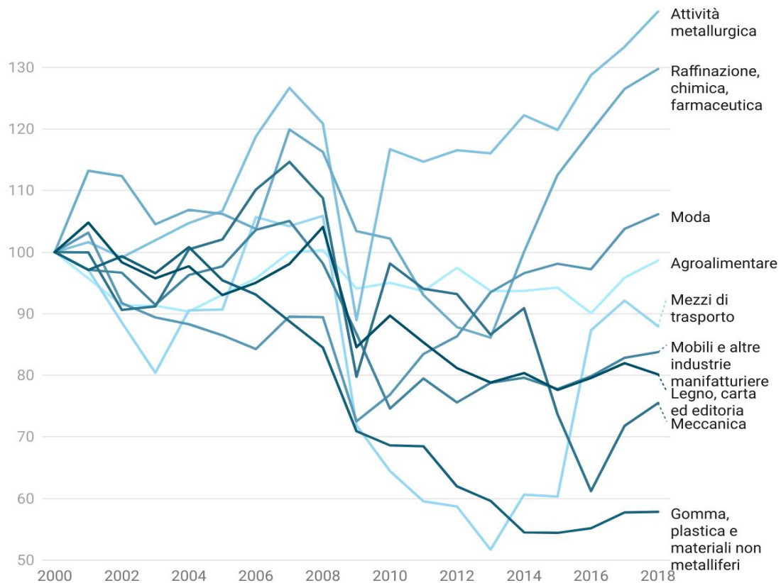
Grafico 2. PRODUZIONE. NUMERO INDICE 2000=100
