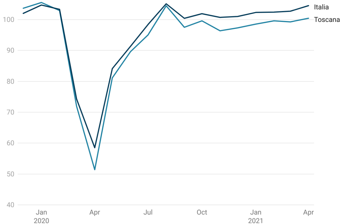
Grafico 7. PRODUZIONE. NUMERO INDICE 2015=100
